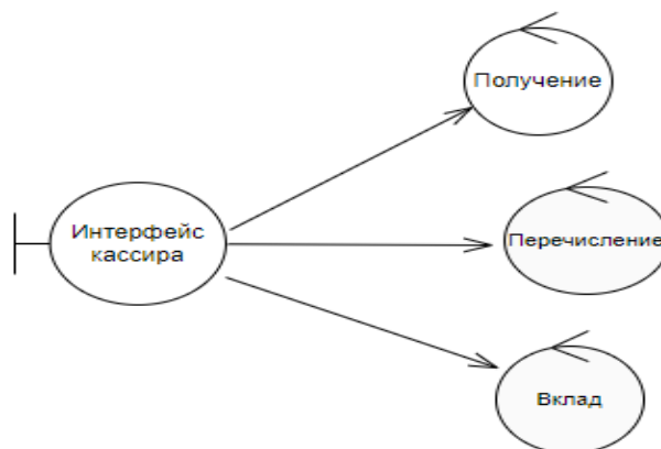
Рисунок 11. Отношение (направленной) ассоциации
