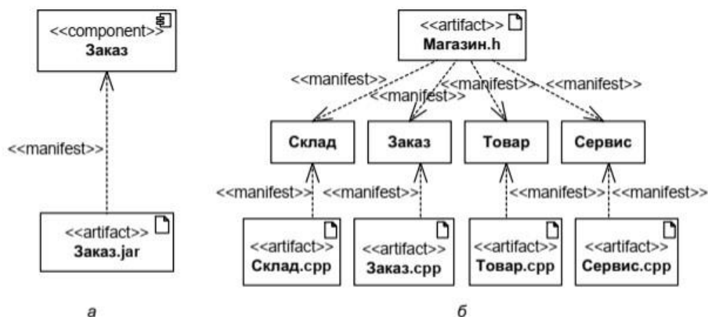
Рисунок 70. Примеры изображения отношения манифестации: а – между артефактов и компонентом; б – между артефактами, компонентами и классами
