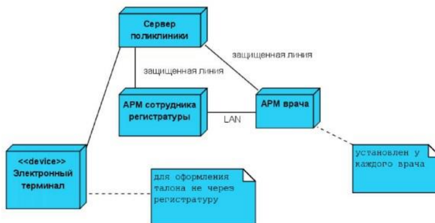
Рисунок 73. Диаграмма развертывания для системы «Поликлиника»
