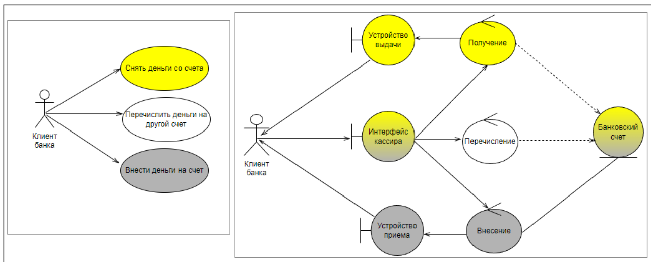
Рисунок 23. Реализация каждого из вариантов использования (слева), в структуре классов анализа (справа)
