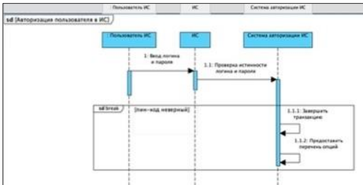
Рисунок 32. Диаграмма последовательности для описания процесса авторизации пользователя в информационной системе с использованием оператора break
