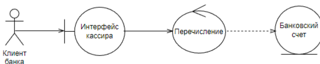
Рисунок 20. Реализации варианта использования «Перечислить деньги на другой счет» в диаграмме классов анализа
