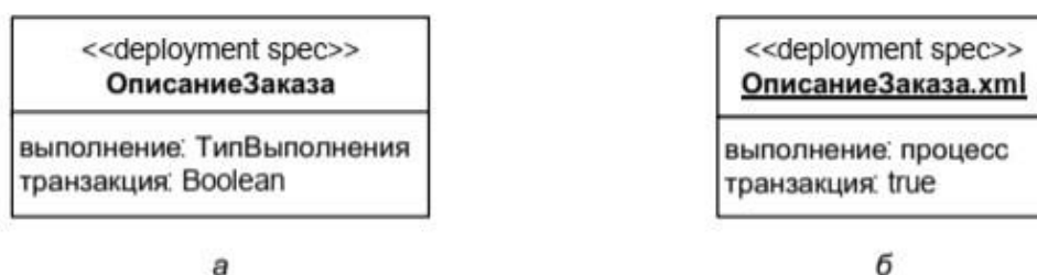
Рисунок 67. Примеры изображения спецификации развертывания для артефакта: а – уровня типа; б – уровня экземпляра
