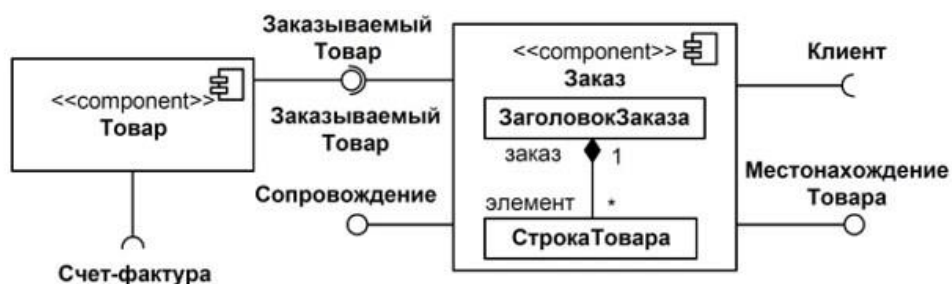
Рисунок 55. Пример изображения компонентов с интерфейсами
