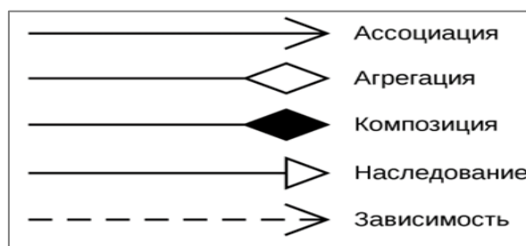
Рисунок 10. Виды отношений между классами анализа
