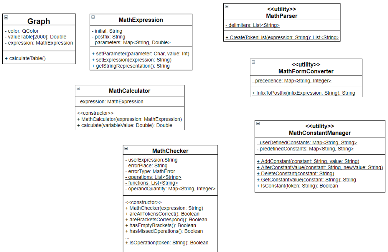
Рисунок 44. Классы с атрибутами и операциями
