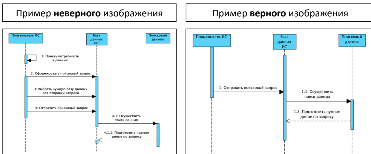
Рисунок 37. Примеры верного и неверного распределения действий (или поведения) между объектами
