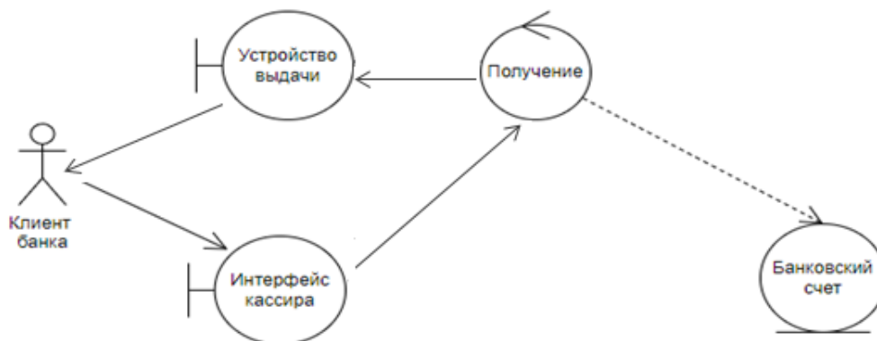
Рисунок 18. Реализации варианта использования «Снять деньги со счета» в диаграмме классов анализа
