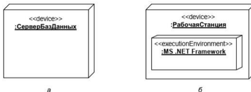
Рисунок 65. Примеры изображения: а – простого устройства; б – устройства контейнера
