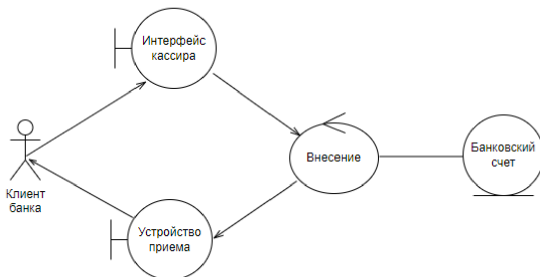
Рисунок 22. Реализации варианта использования «Внести деньги на счет»
