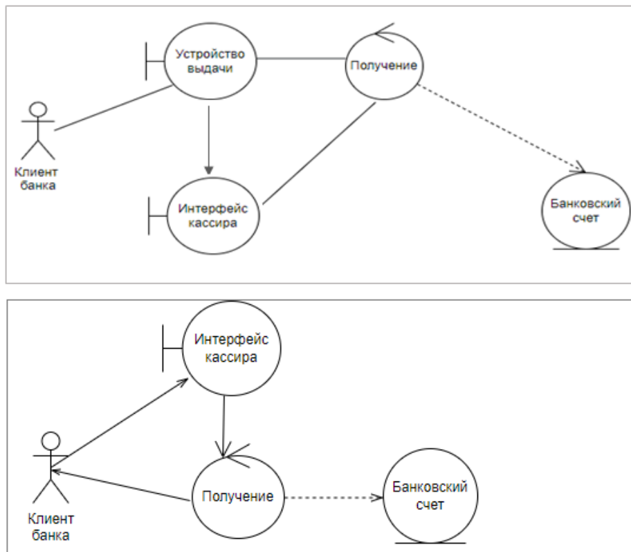
Рисунок 18а. Неверные варианты реализации варианта использования «Снять деньги со счета» в диаграмме классов анализа
