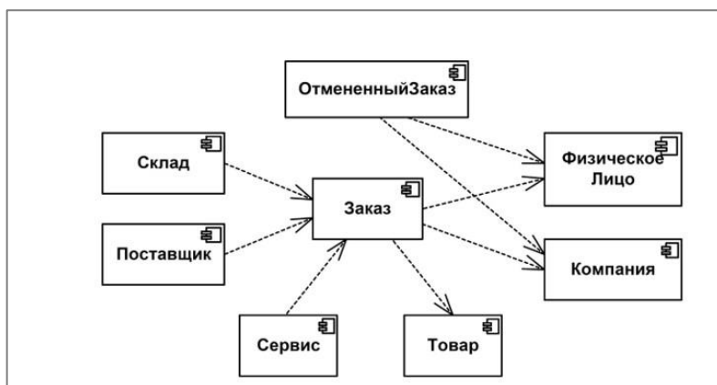
Рисунок 56. Пример отношений зависимости между компонентами
