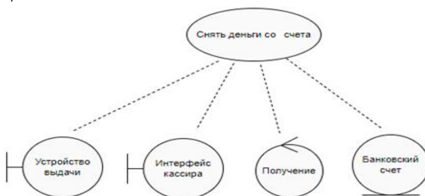
Рисунок 17. Состав классов варианта использования «Снять деньги со счета»
